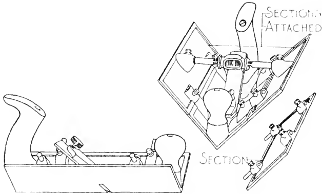
FIG. 80. CORE-BOX PLANE.
